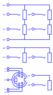
接点示意图
